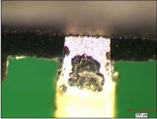
Matte Sn on Cu (optical)
