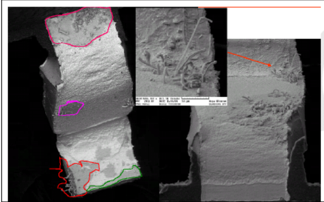
Matte Sn on Cu (SEM)
