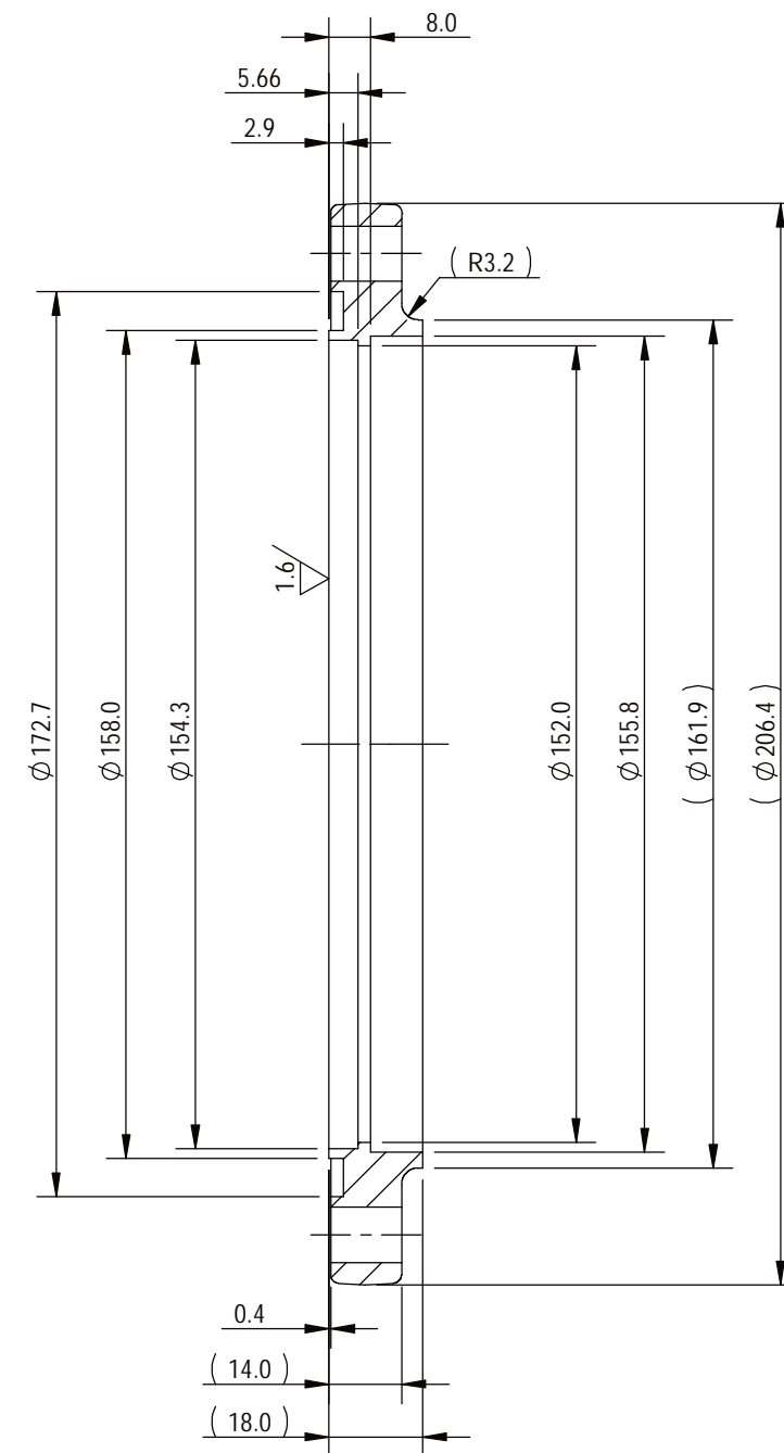
SECTION A-A
