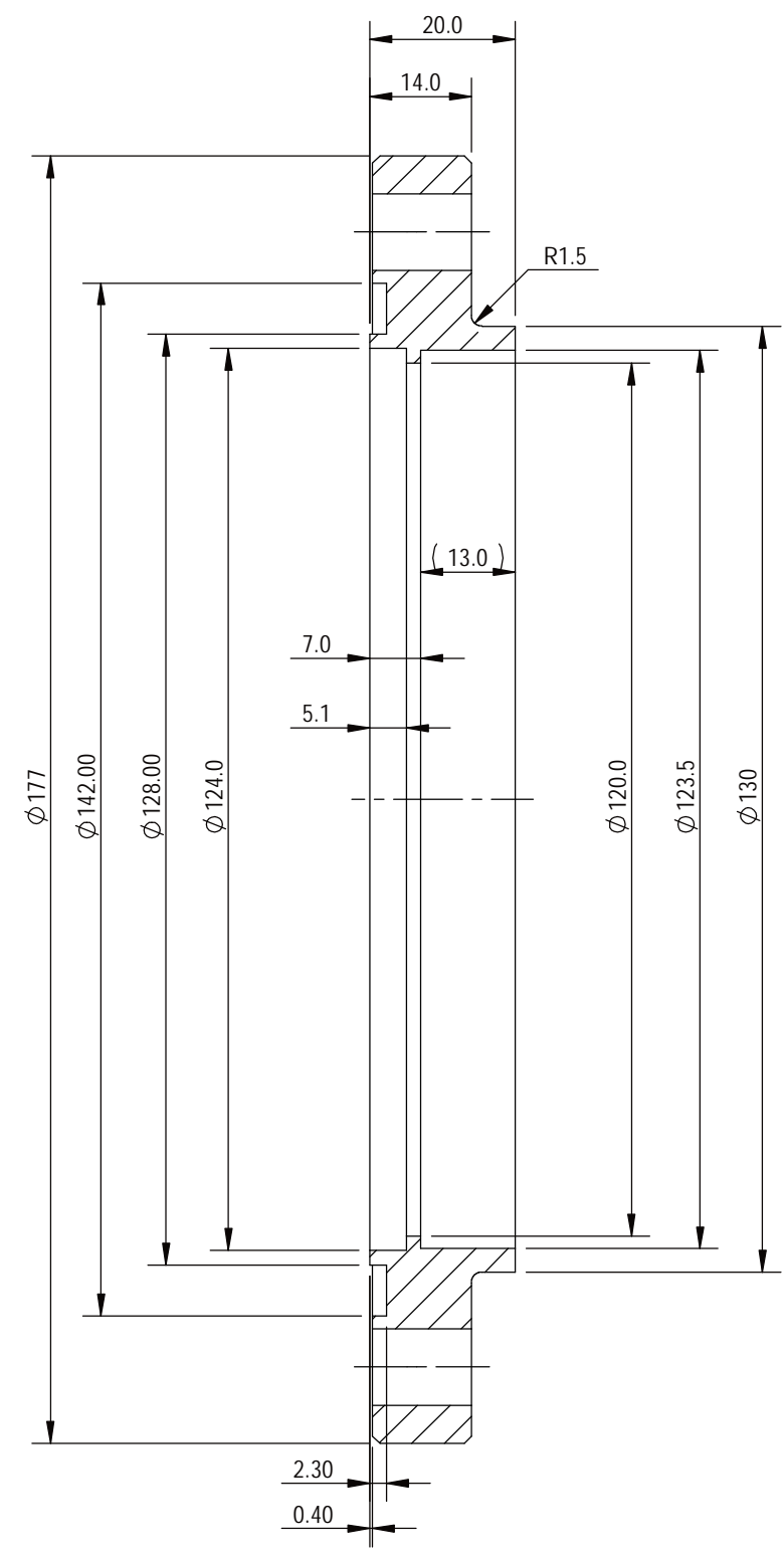
SECTION A-A
