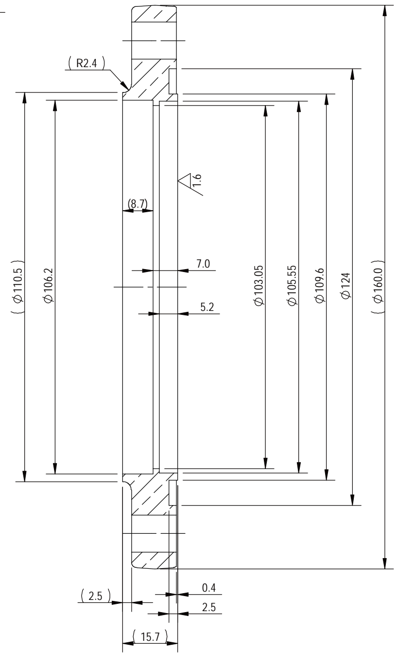
SECTION A-A
