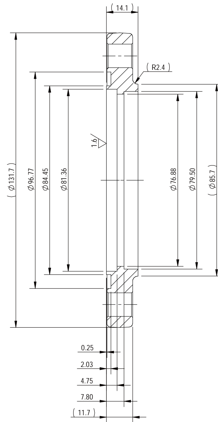
SECTION A-A
